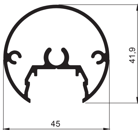
PASAMANOS SKYLINE 10+10 mm. ADR 4034 peso: 0,882 kgrs/mt.
