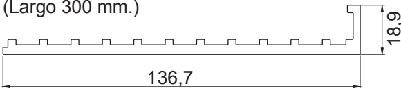
AA 418 Suplemento para AA 411 (Largo 300 mm.)
