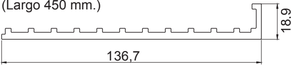
AA 417 Suplemento para AA 410 (Largo 450 mm.)
