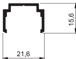
SUPLEMENTO PASAMANOS 8+8 mm. ADR 4035 peso: 0,201 kgrs/mt.
