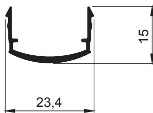
TAPA PASAMOS ADR 4036 peso: 0,170 kgrs/mt.
