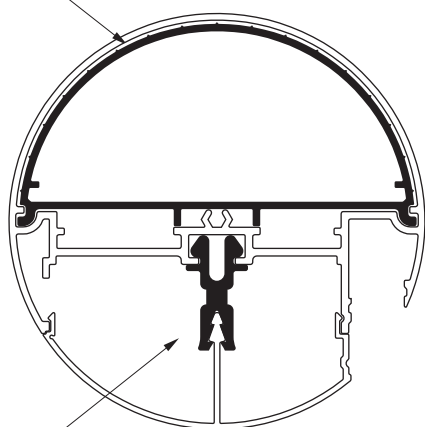
Detalle ubicación Clip AA358-6
