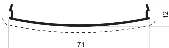
ADR 3012 Tapa Pasamanos Peso: 0,278 kg/m (Baranda reforzada)
